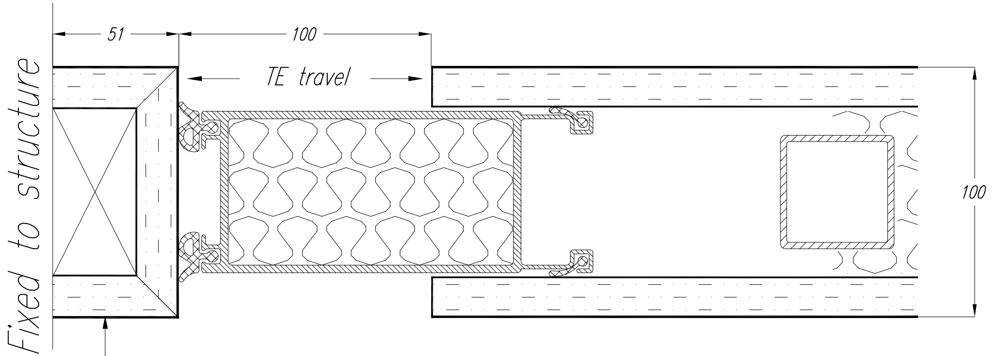
Telescopic Wall Jamb
